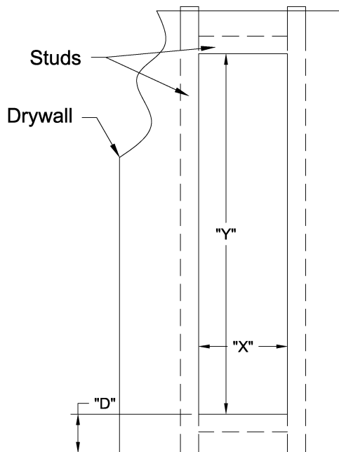
Drywall & Stud Detail
